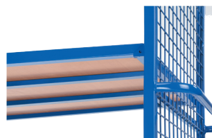
Étagère renforcée. Charge : 100 kg uniformément répartie.
